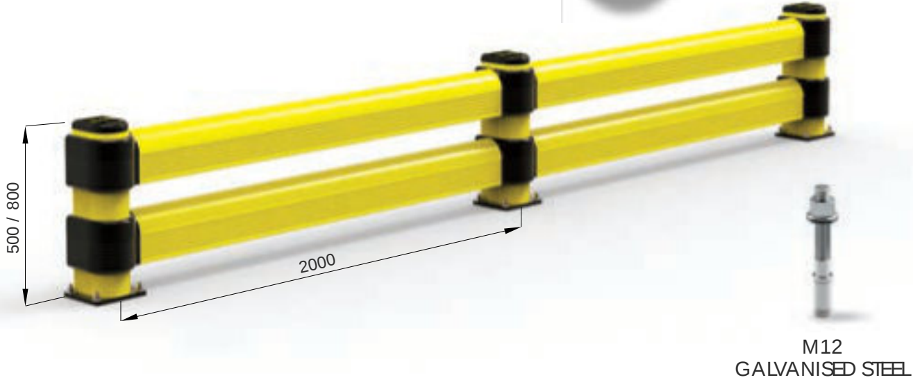
LINK LM 500 800
