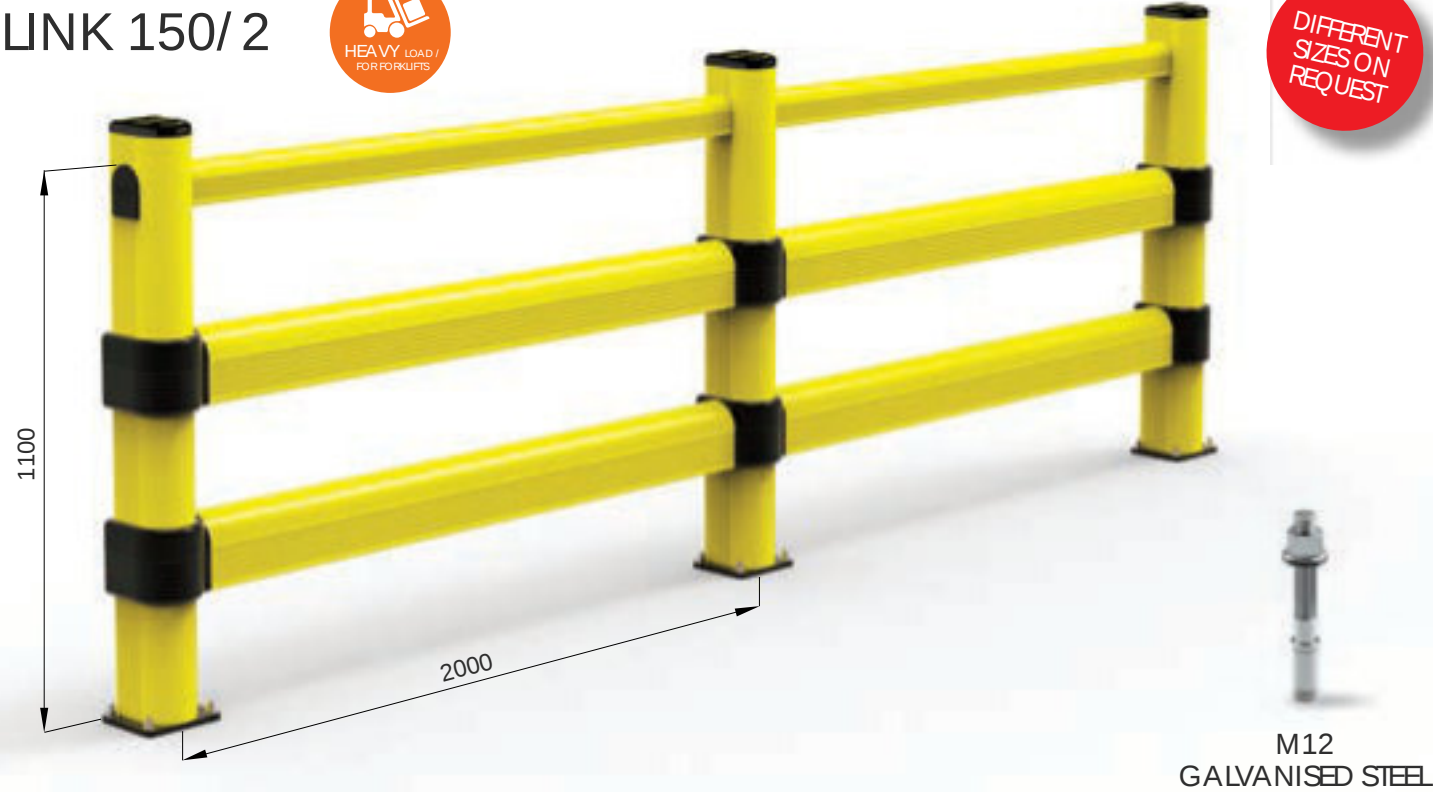
LINK 150/2
