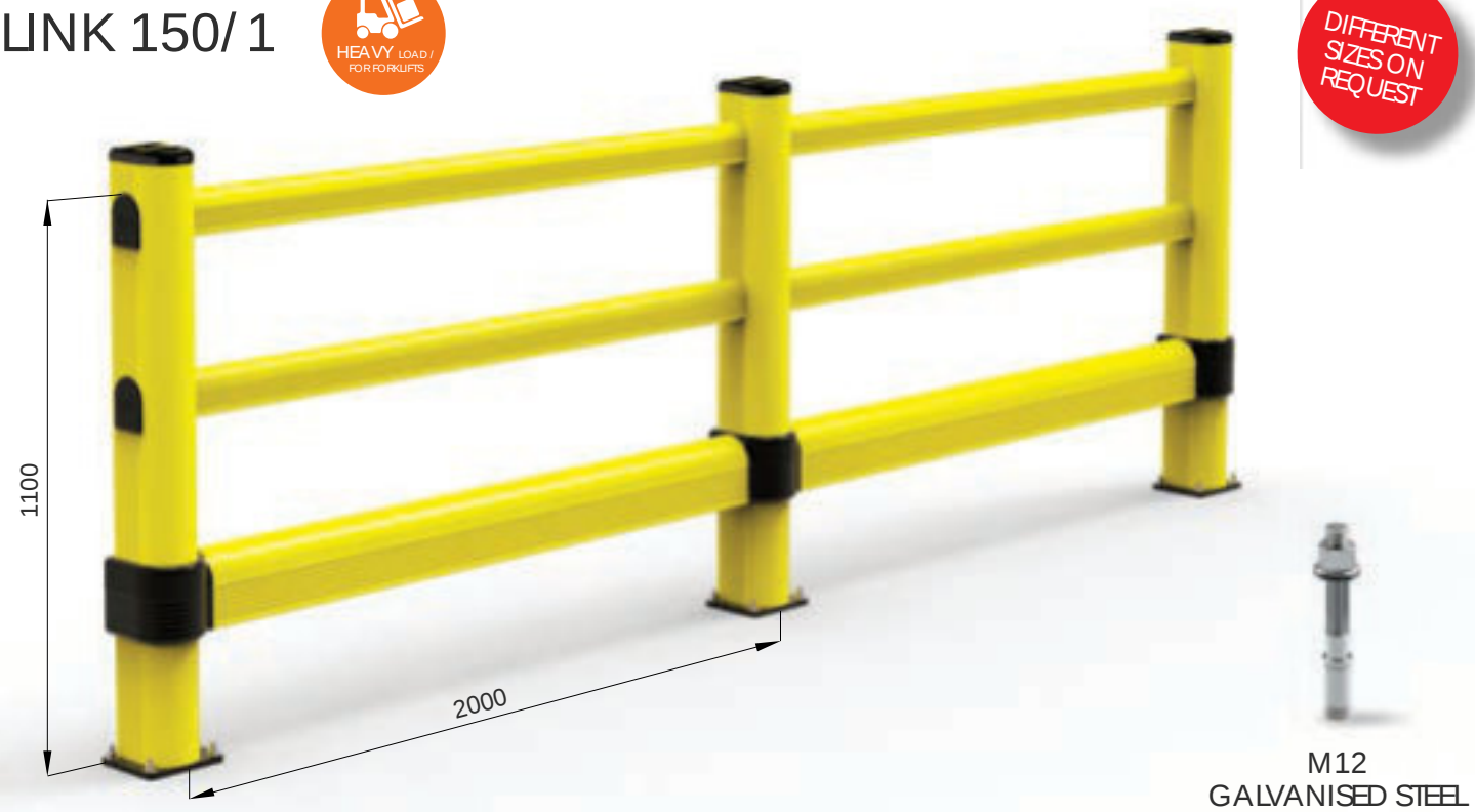
LINK 150/1
